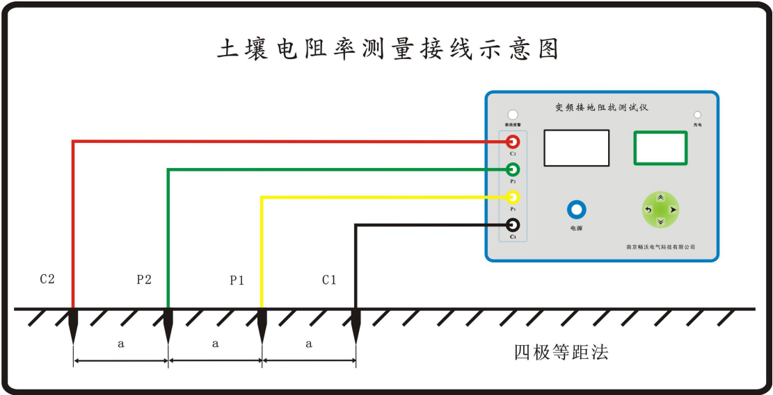
a-电流极与电位极间距；C1、C2-电流极；P1、P2-电位极
