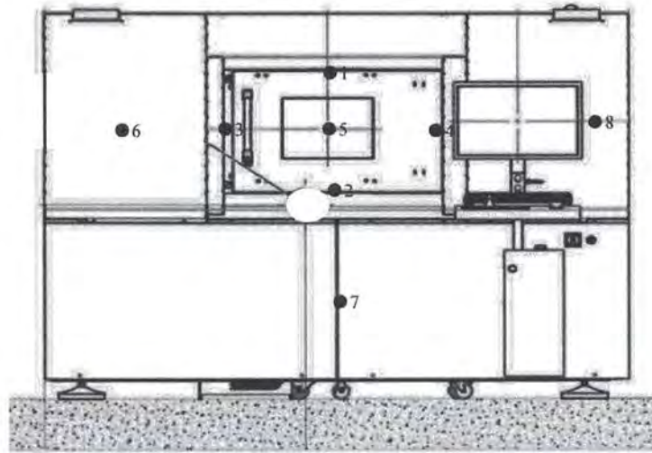
主视图
