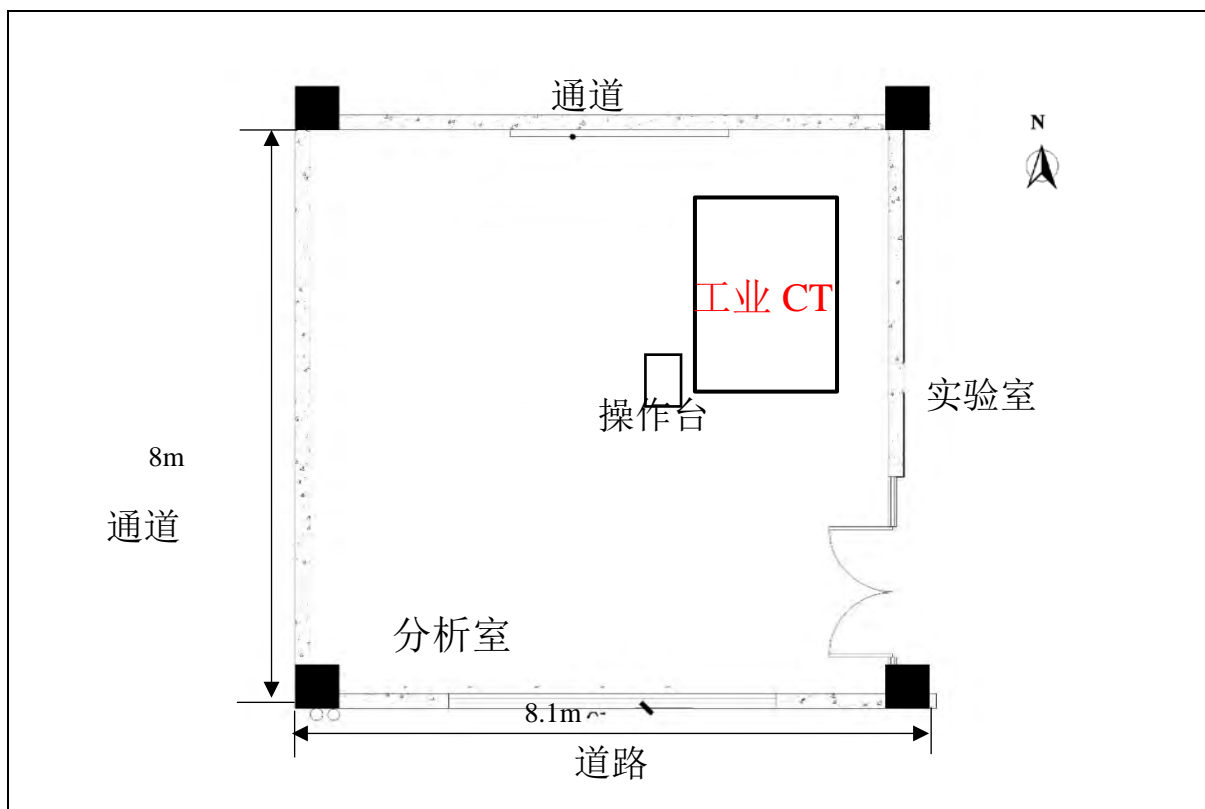
图 6-2 工业 CT 四周场所分布图
