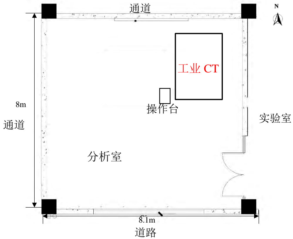
图 3-2 工作场所布置图
