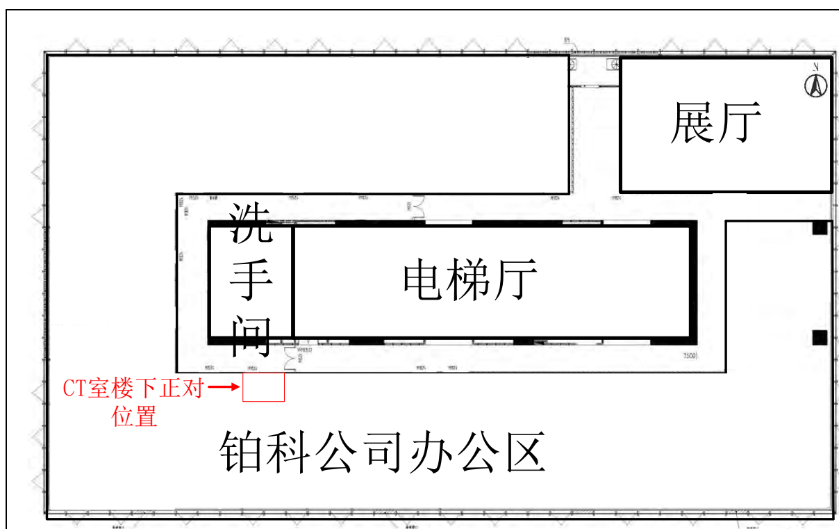
图 2-3 B 座 13 层平面图
