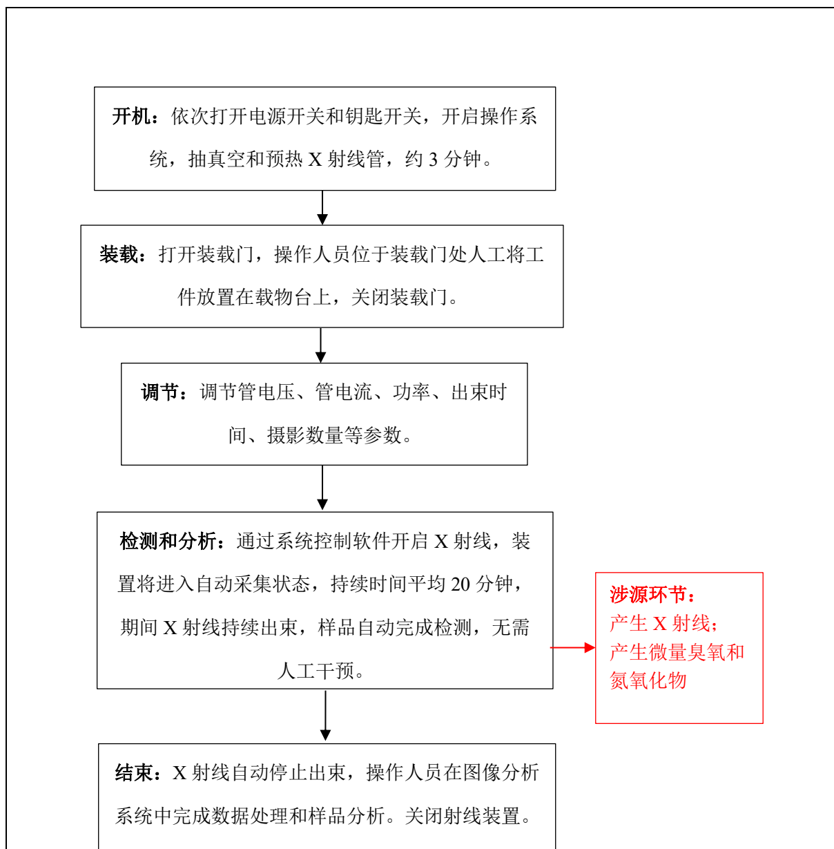
图 2-8 操作流程和产污环节图
