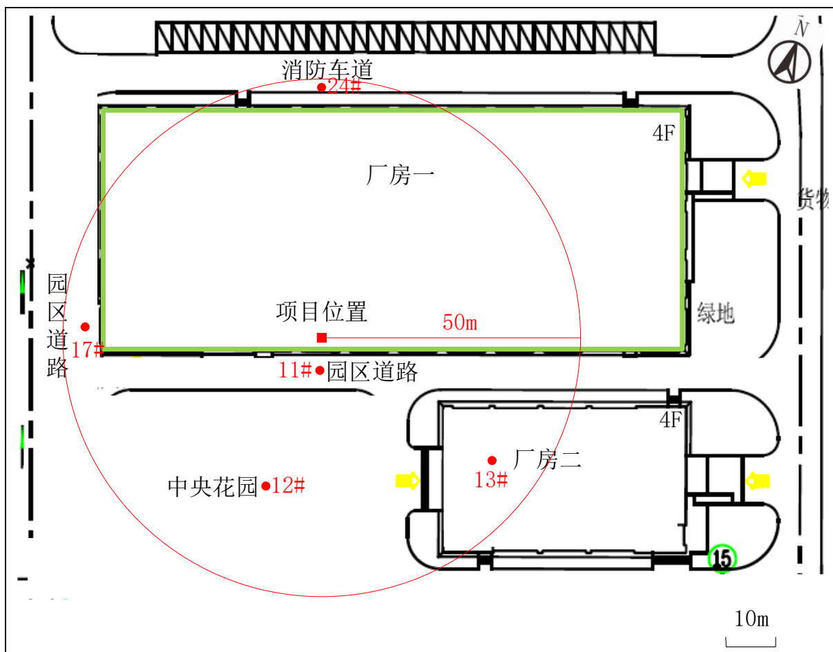
图 8-5 项目 50m 范围检测布点图
