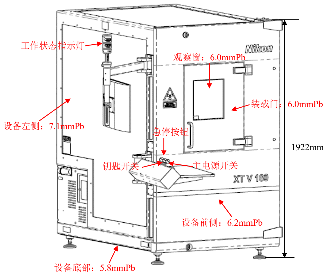
图 10-1 工业 CT 侧视图
