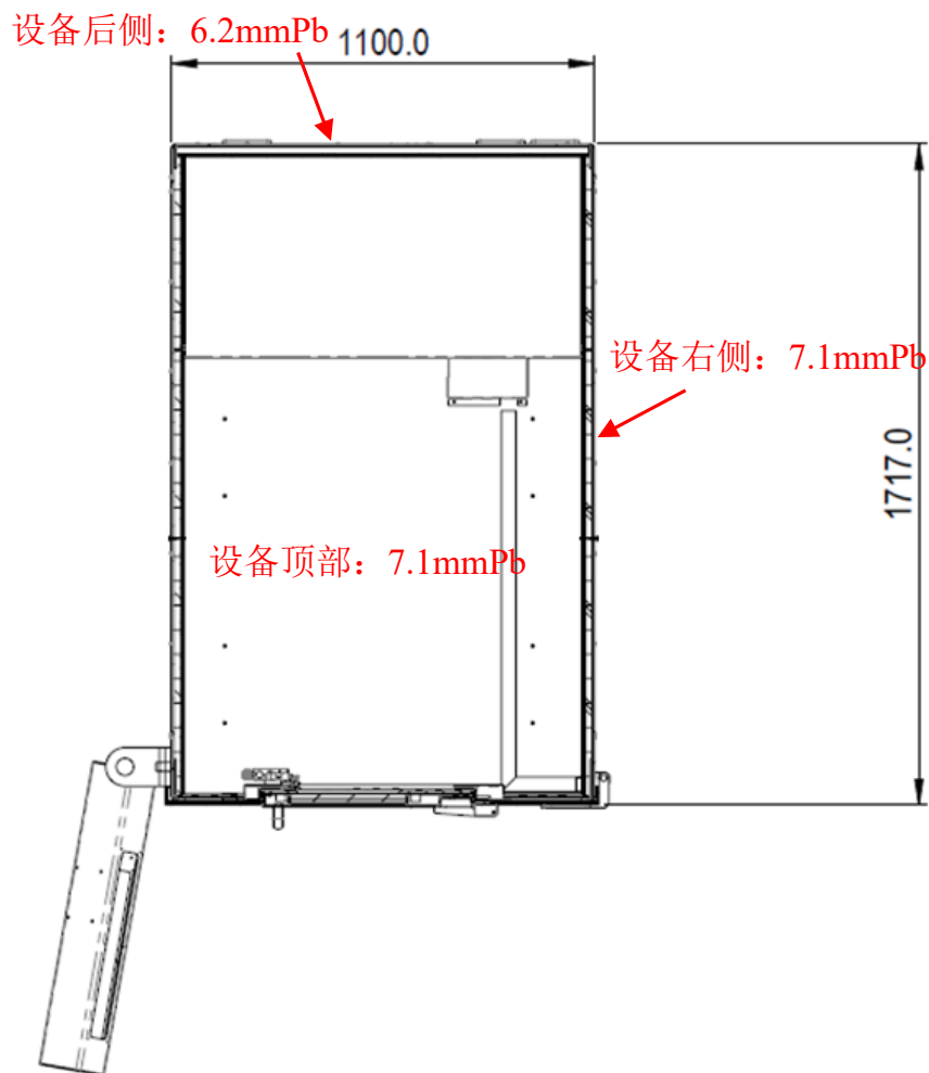
图 10-2 工业 CT 俯视图
