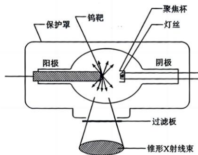
图 9-3 X 射线管示意图
