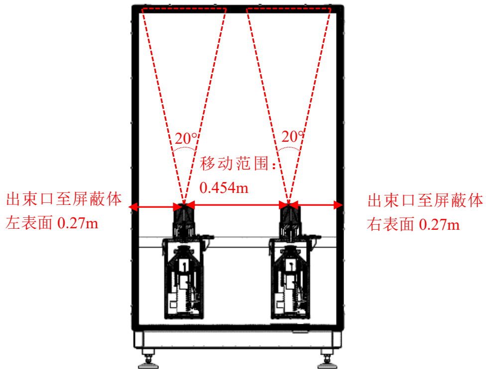
图 11-1.2 射线发生器分布示意图（正视）
