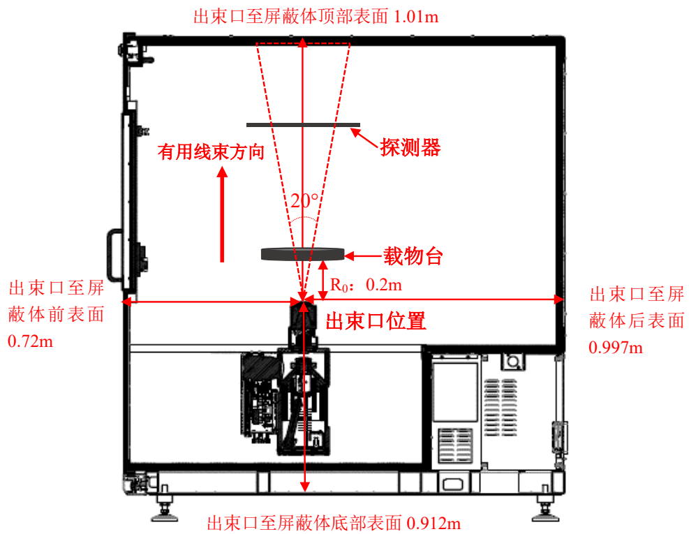
图 11-1.1 射线发生器分布示意图（右视）
