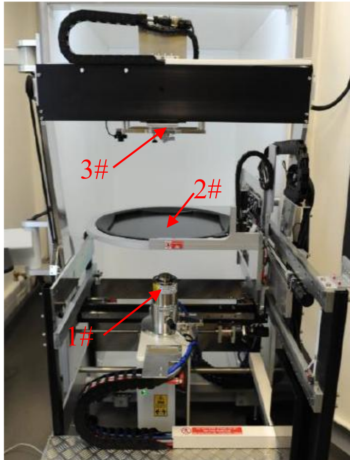
图 9-2 工业 CT 内部结构图
