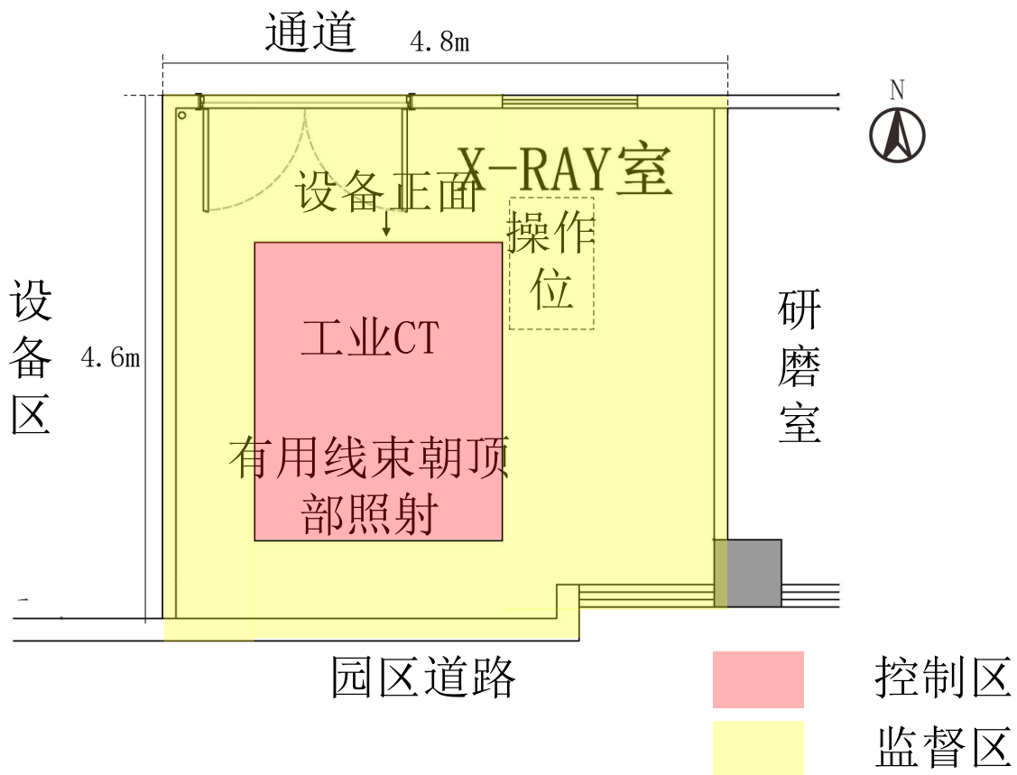
图 10-6 辐射工作场所布局和分区示意图
