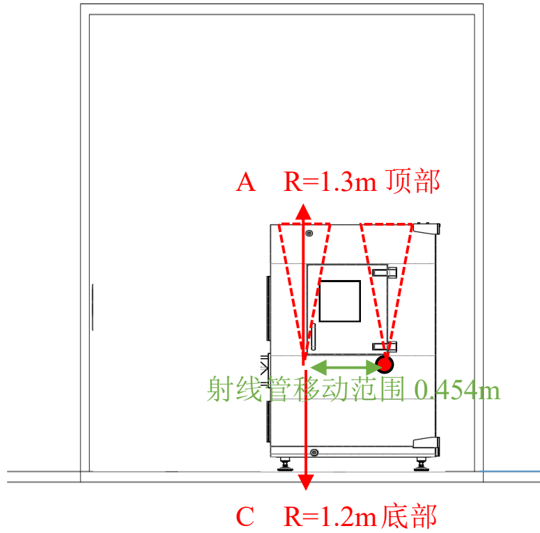
图 11-2.1 关注点分布示意图 (立面)
