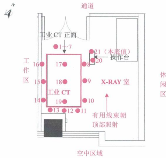
附图 1: 检测布点图
