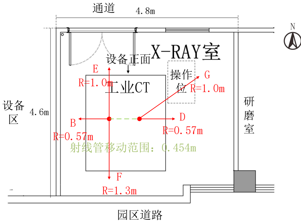
图 11-2.2 关注点分布示意图 (平面)
