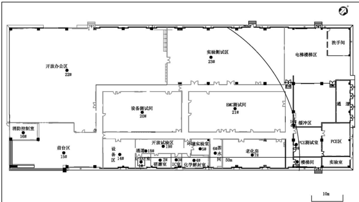
图 8-3 1层检测布点图
