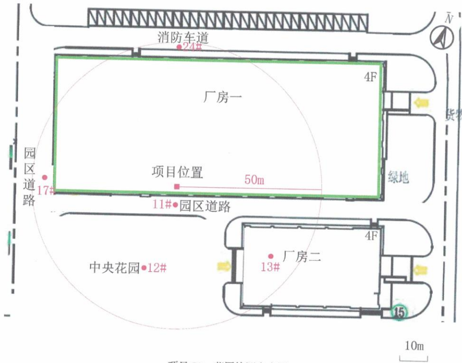
项目 50m 范围检测布点图
