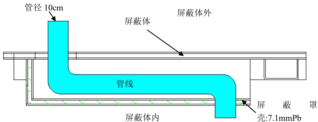
图 10-3 管线穿屏蔽体示意图
