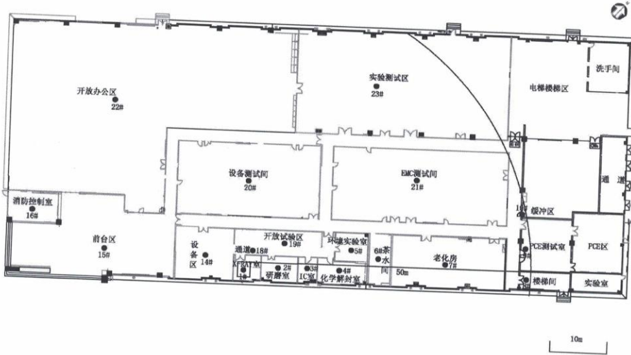
1层检测布点图
