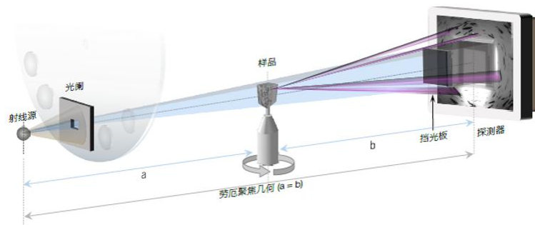
图 9-4 工业 CT 工作原理示意图
