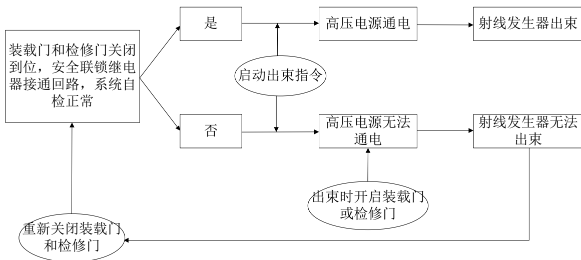
图 10-4 门机联锁逻辑图
